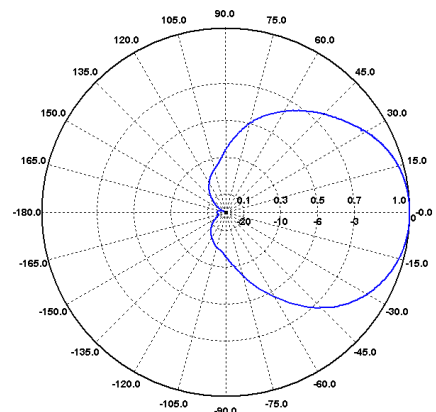
H-Ebene / H-Plane 700 MHz
